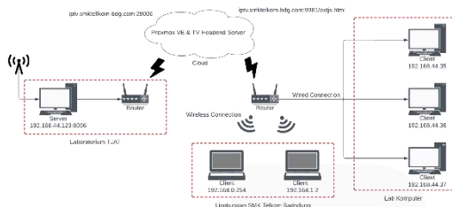
Gambar 9 (Model Miniatur)
