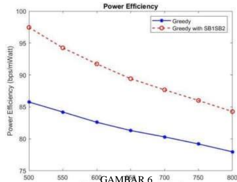
GAMBAR 6 HASIL SIMULASI EFISIENSI DAYA
