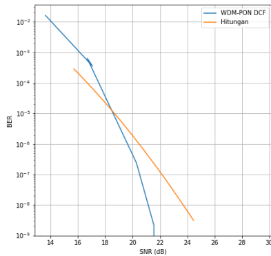
GAMBAR 17. Hasil WDM-PON DCF
