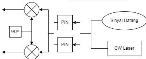
GAMBAR 2. Arsitektur Deteksi Koheren
