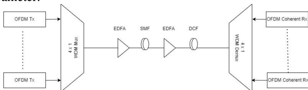
GAMBAR 8. Koheren WDM Kabel SMF dan DCF
