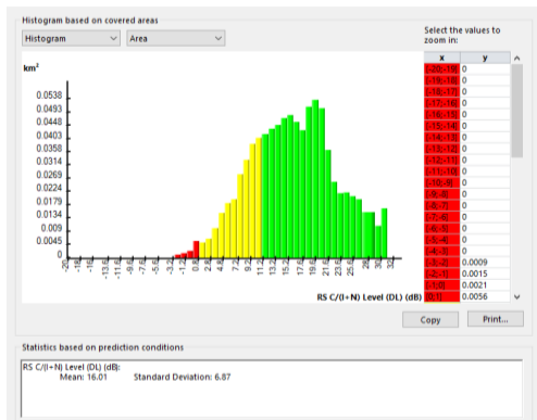
Gambar 12 Nilai SINR menggunakan skenario I
