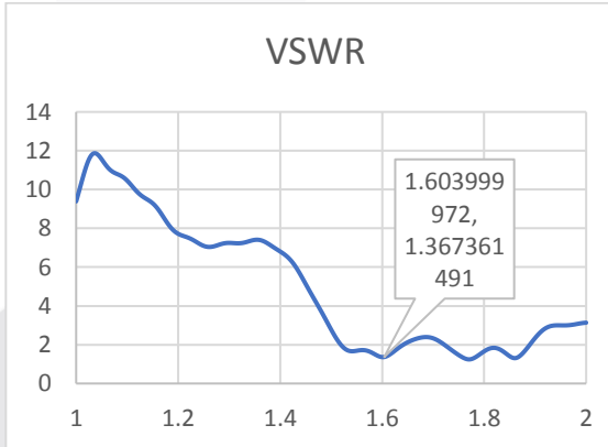
GAMBAR 4 NILAI VSWR PENAMBAHAN SLOT SETELAH OPTIMASI.
