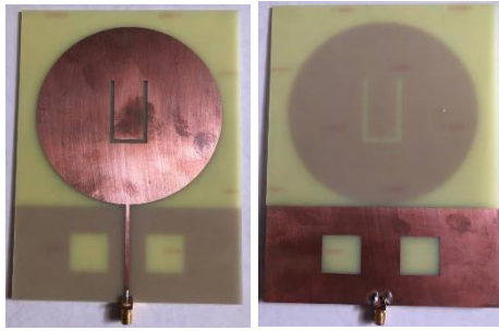
GAMBAR 11. REALISASI ANTENA
