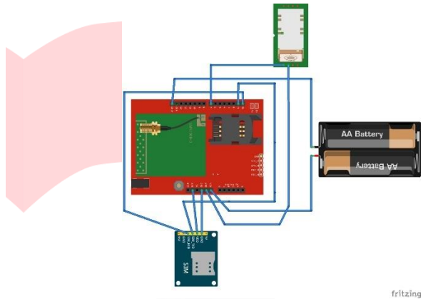
GAMBAR 3.4 SKEMATIK RANGKAIAN
