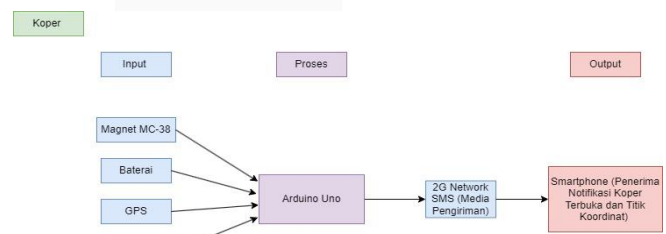
GAMBAR 3.1 BLOK DIAGRAM SISTEM UTAMA
