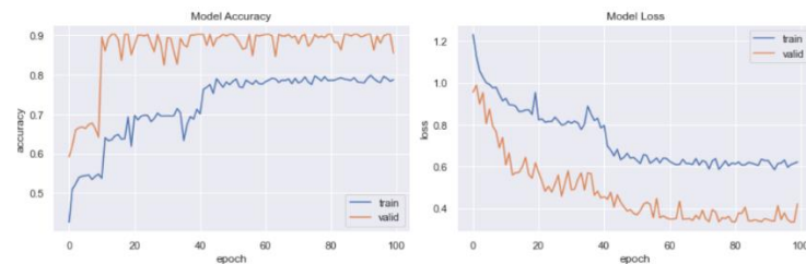
GAMBAR 7 GRAFIK AKURASI DAN LOSS MODEL CNN MODIFIKASI
