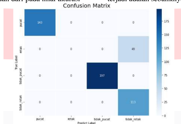
GAMBAR 8 CONFUSION MATRIX MODEL CNN MODIFIKASI
