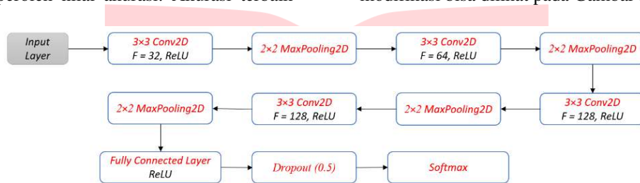
GAMBAR 5 DIAGRAM ARSITEKTUR CNN MODIFIKASI
