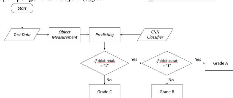
GAMBAR 6 DIAGRAM ALIR MESIN PREDIKSI
