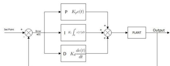
Gambar 3 Blok Diagram Kontroler PID
