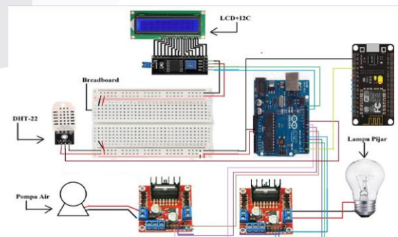
GAMBAR 2 Rancangan Rangkaian Elektronik
