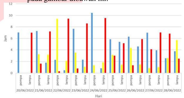
GAMBAR 8 Data Penggunaan Aktuator tanggal 20-28 Juni 2022
