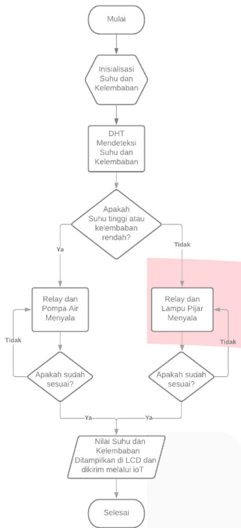
GAMBAR 3 Diagram Alir Sistem
