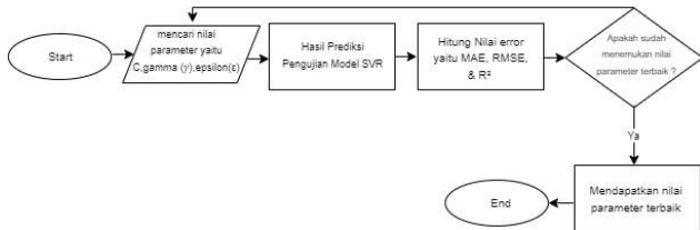
GAMBAR 3. 5 DIAGRAM ALIR MENDAPATKAN ANGKA PARAMETER TERBAIK DENGAN ALGORITMA GRID SEARCH
