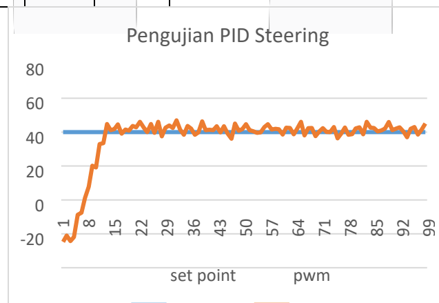
Gambar 4.1. Pengujian PID Steering
