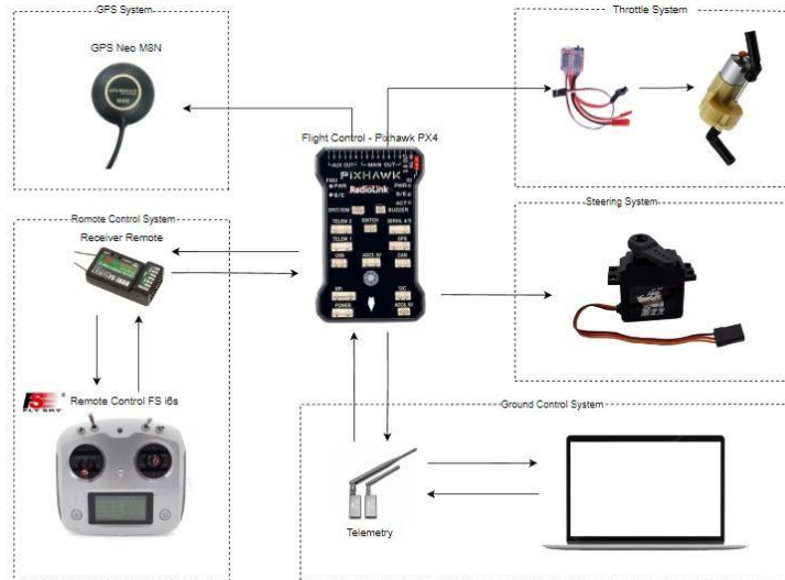
Gambar 3.1 Desain Perangkat Keras
