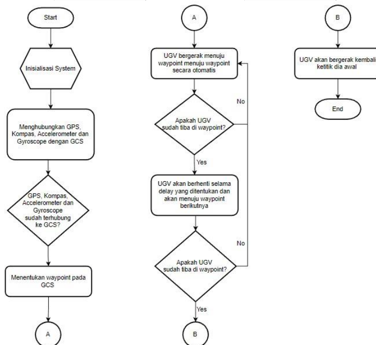
Gambar 3.2. Diagram Alir
