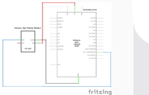
GAMBAR 2.2 Skematik Rangkaian Sensor Api Flame
