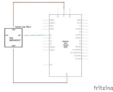
GAMBAR 2.3 Skematik Rangkaian Sensor Gas MQ-2
