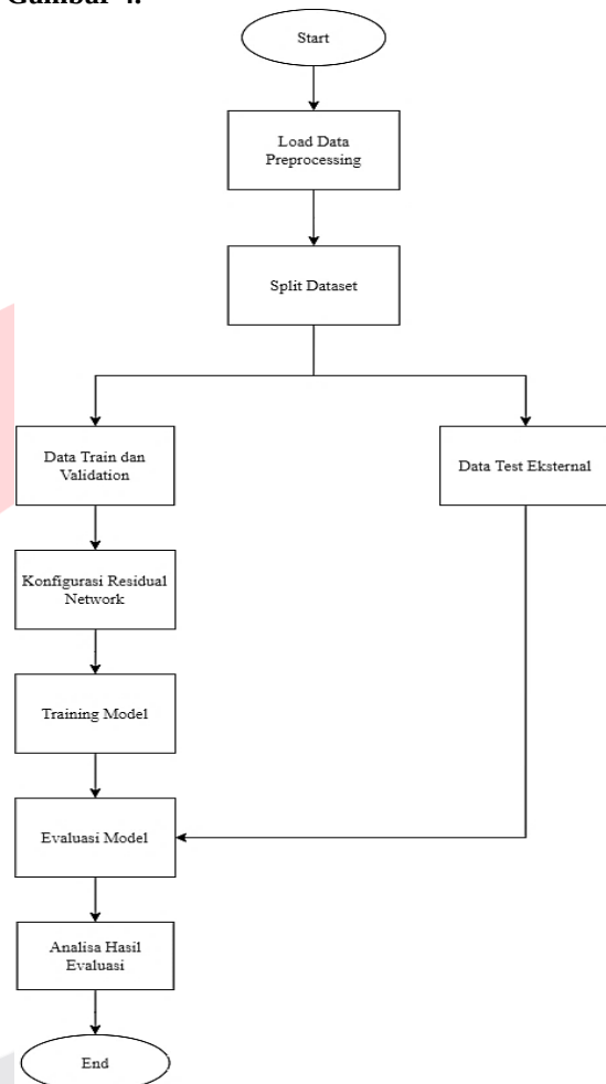
GAMBAR 4. Flowchart Klasifikasi
