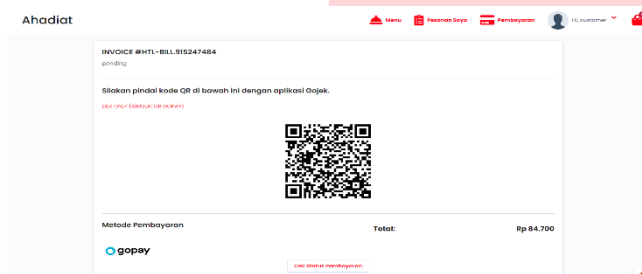
GAMBAR 9 IMPLEMENTASI PEMBAYARAN
