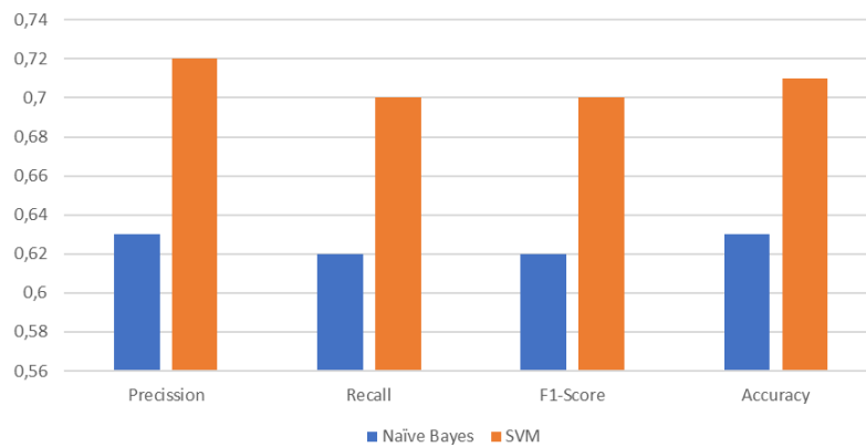
Gambar 11. Diagram Perbandingan SVM dan NB (50/50)
