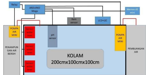
Gambar 4 Rancangan mekanisme keseluruhan
