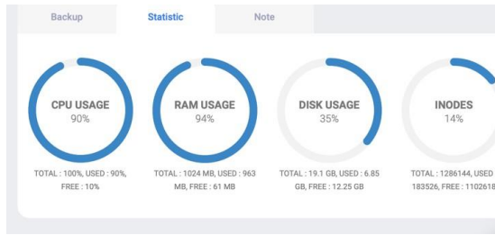
Gambar 4- 19 Statistik VPS setelah diserang
