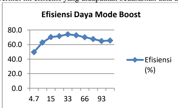
Gambar 4.6 Grafik Efisiensi Daya Mode Boost
