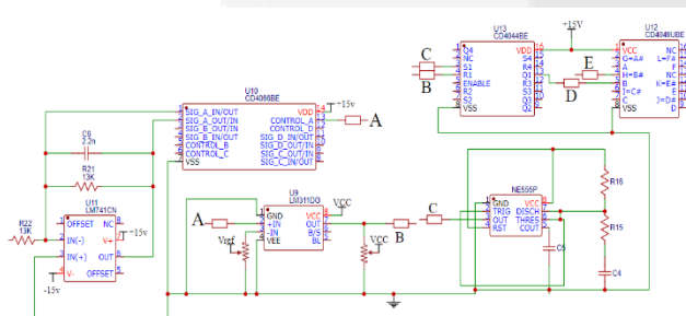
Gambar 3. 6 Wiring diagram Rangkaian Kendali Satu Siklus
