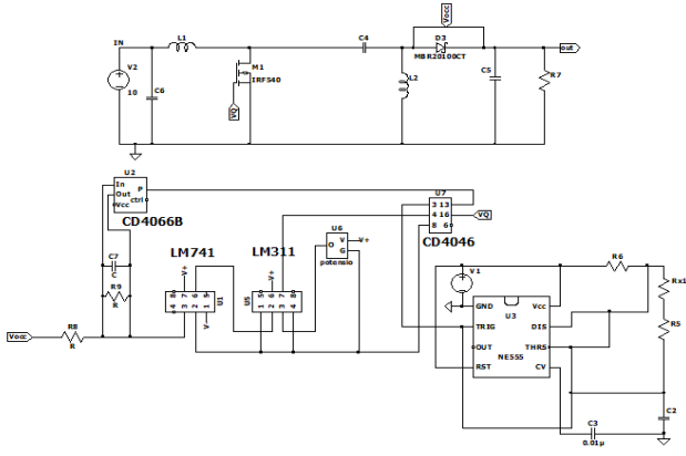
Gambar 3.1 Desain Sistem
