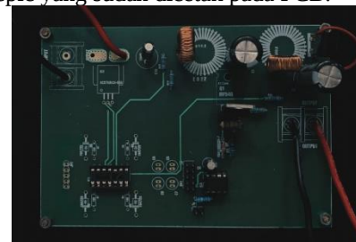
Gambar 3. 4 PCB Konverter Sepic
