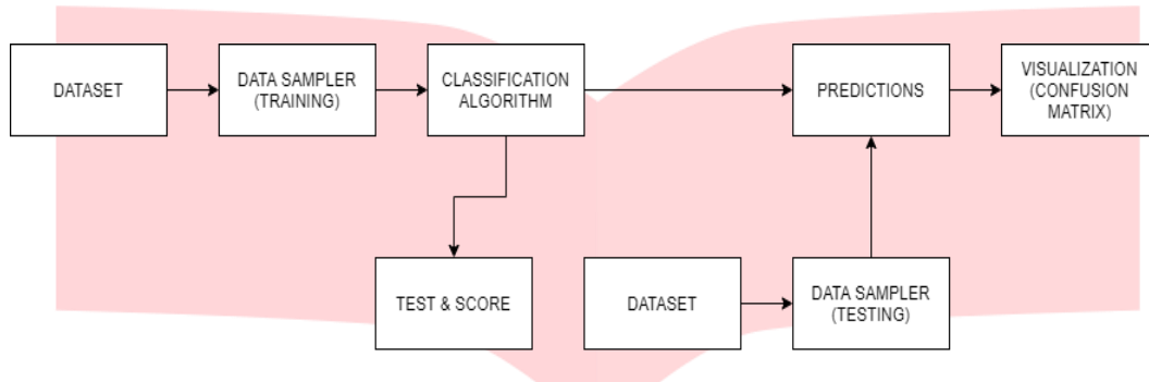
Gambar 6. Tahap Klasifikasi Menggunakan Orange Data Mining
