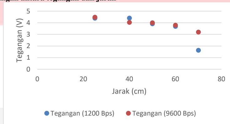
Gambar 1 Grafik perbandingan tegangan dan jarak pada sudut 0°
