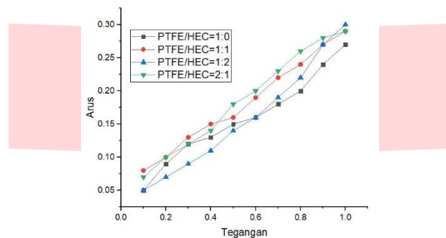
Gambar 3.3 Grafik V-I Variasi komposisi binder .
