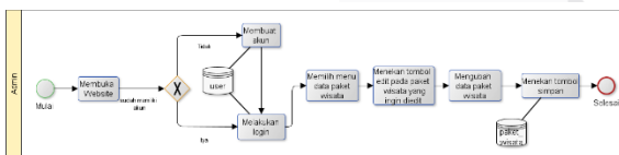
Gambar 3 - 4 BPMN Usulan Mengedit Paket Wisata Haji dan Umrah
