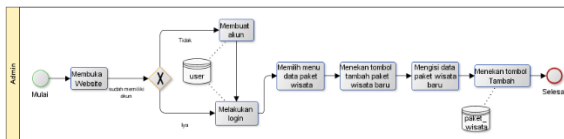
Gambar 3 - 3 BPMN Usulan Tambah Paket Wisata Haji dan Umrah
