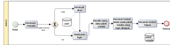
Gambar 3 - 5 BPMN Usulan Hapus Paket Wisata Haji dan Umrah
