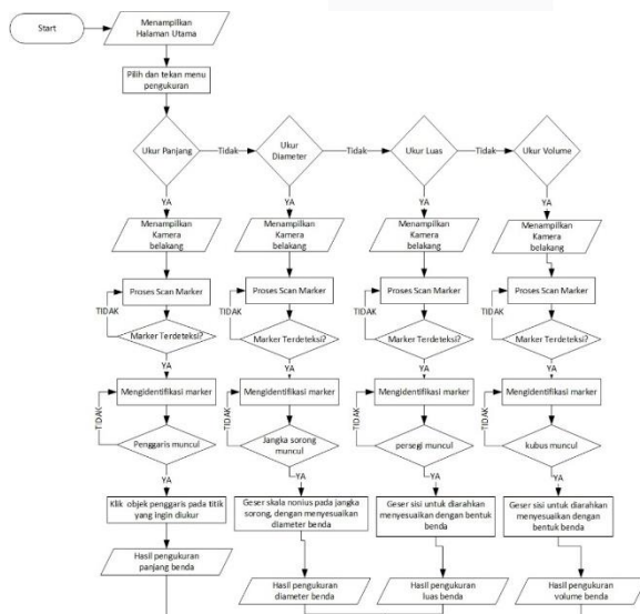
Gambar 3. 2 Flowchart Aplikasi
