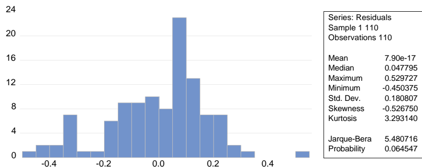
Gambar 2 Jarque-Bera Test
