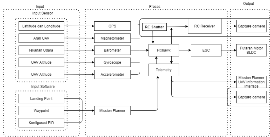
Gambar 2. Desain Sistem
