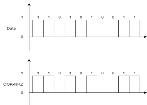
Gambar 2. 2. Modulasi OOK
