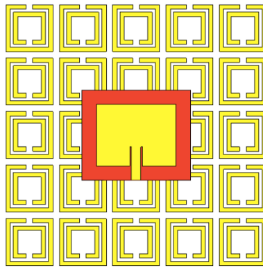
Gambar 3.3 Struktur metamaterial 5 x 5 yang ditambahkan sebagai reflektor
