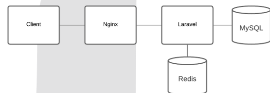
Gambar 1 Arsitektur Aplikasi Web Service
