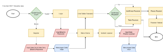
Gambar 2. 4 Flowchart MVP Penyedia Jasa
