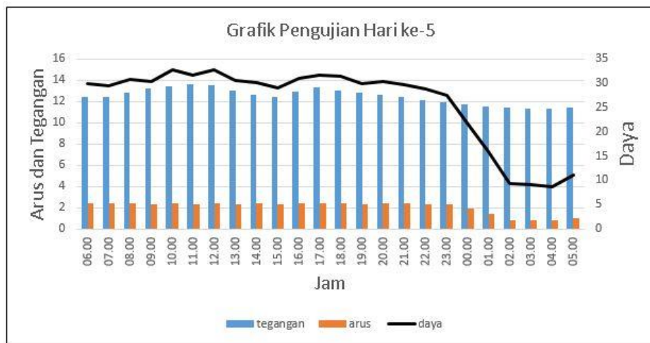
Gambar 4. 5 Grafik pengujian hari ke-5
