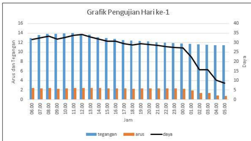
Gambar 4. 1 Grafik pengujian hari ke-1
