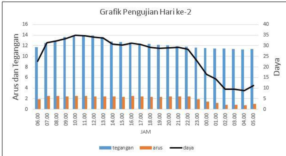
Gambar 4. 2 Grafik pengujian hari ke-2
