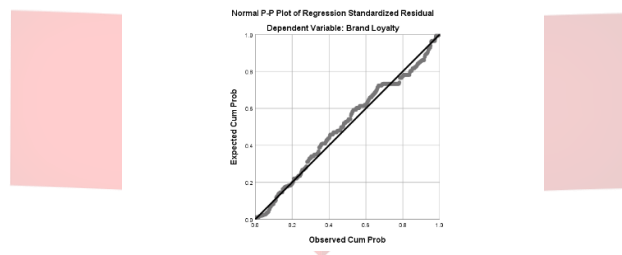
Gambar 1 Grafik P-Plot
