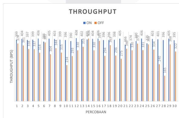
Gambar 4.4 Grafik Throughput Alat menuju Web Service
