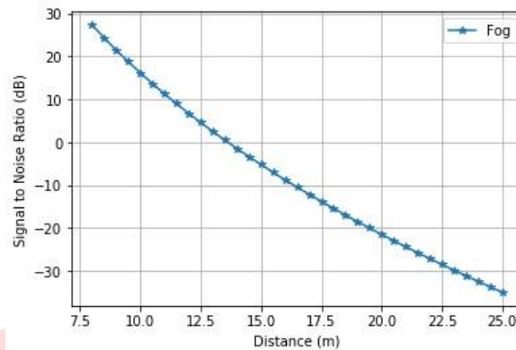
Gambar 9. SNR Skenario 3
