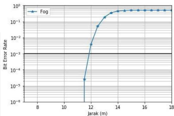
Gambar 10. BER Skenario 3
