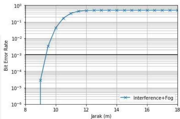
Gambar 12. BER Skenario 4
