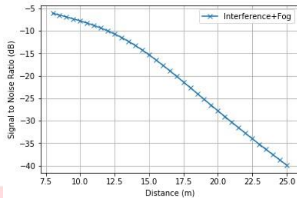
Gambar 11. SNR Skenario 4
