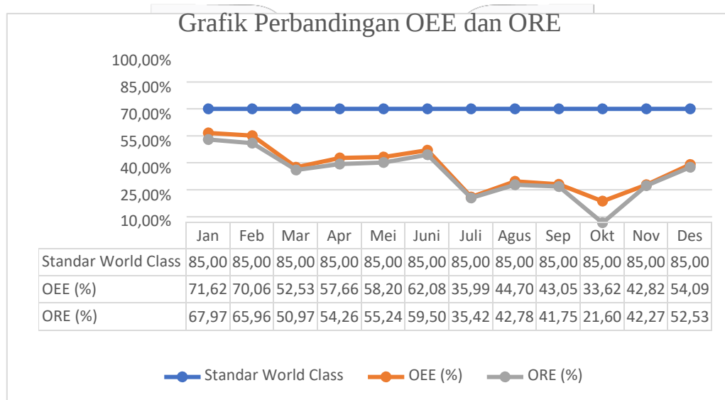
Gambar 3 Grafik Perbandingan OEE dan ORE
