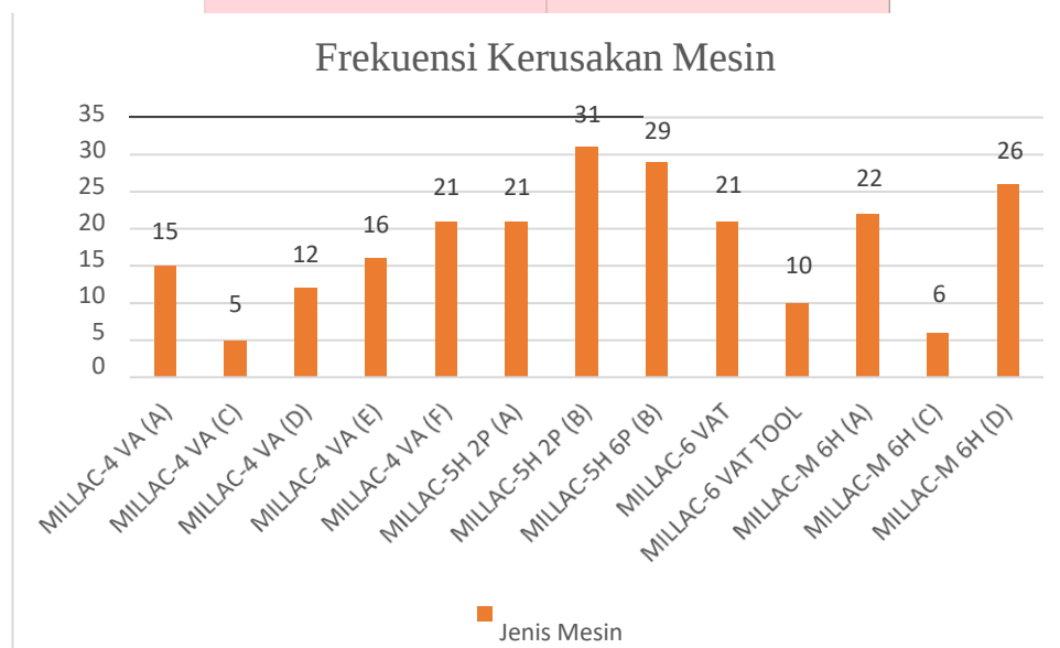
Gambar 1 Data Frekuensi Kerusakan Mesin CNC Millac
