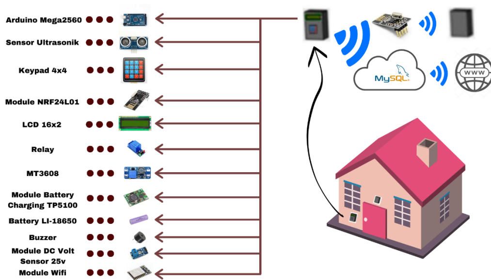
Gambar 3.1 Desain sistem
