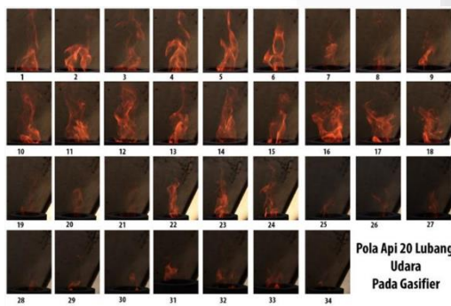
Gambar 9. Pola Api 20 Jumlah Lubang Udara Pada Gasifier
