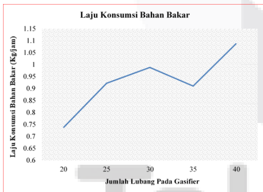
Gambar 3. Grafik Laju Konsumsi Bahan Bakar (FCR)
