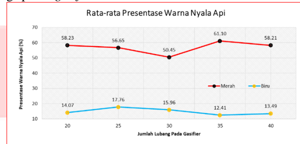
Gambar 5. Grafik Presentase Warna Nyala Api
