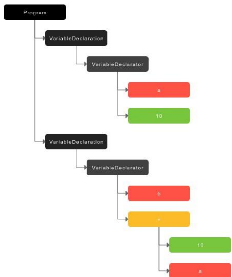
Gambar 1. Visualisasi kode JavaScript menjadi AST
