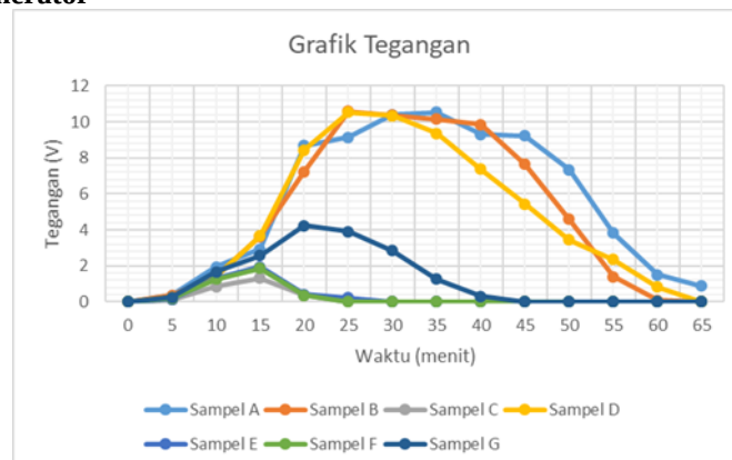
Gambar 5 Grafik Tegangan
