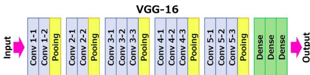
Gambar 7. Arsitektur VGG16
