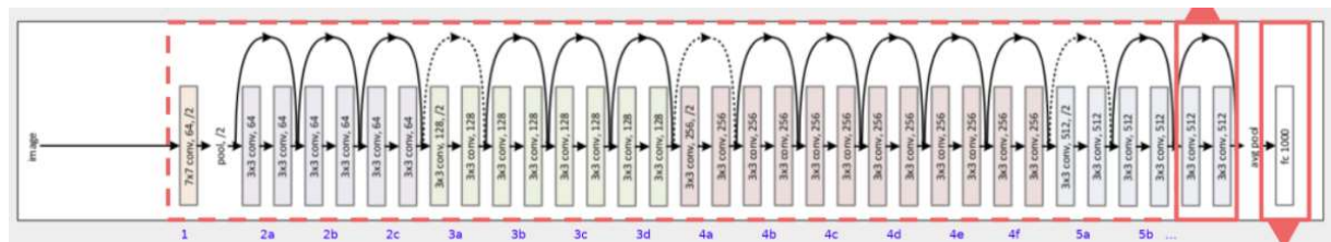
Gambar 9. Arsitektur ResNet50
