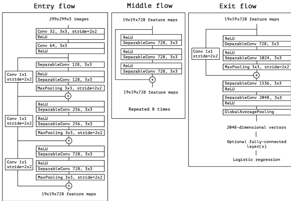
Gambar 10. Arsitektur Xception
