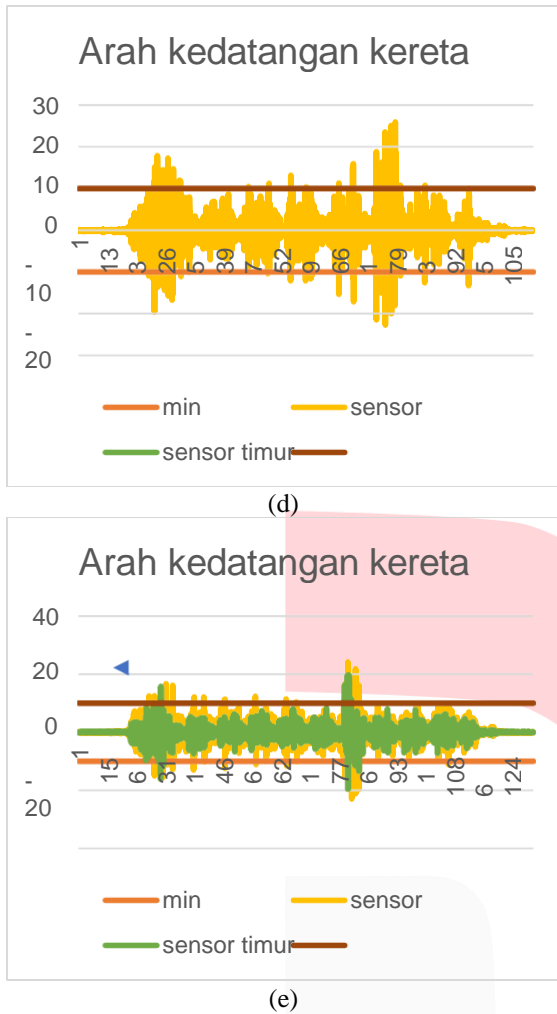
Gambar 4.1 pengujian kedua sensor MPU6050 pada arah kedatangan kereta arah 1
