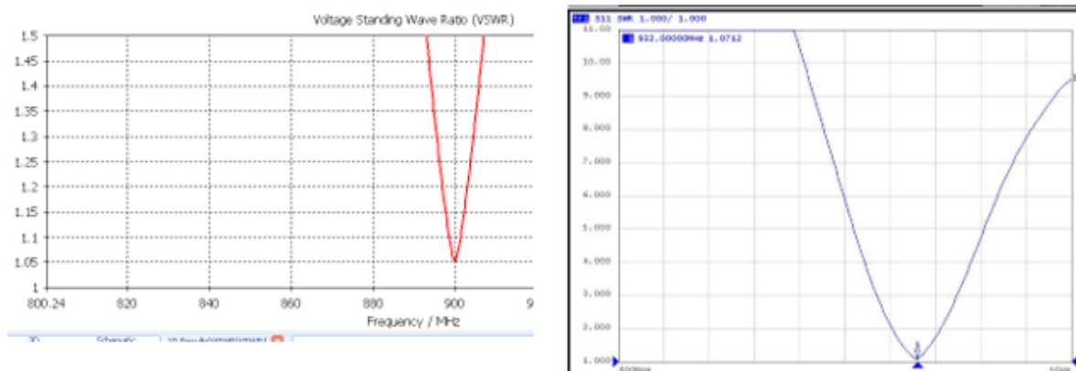
Gambar 11. Hasil perbandingan VSWR simulasi dan pengukuran
