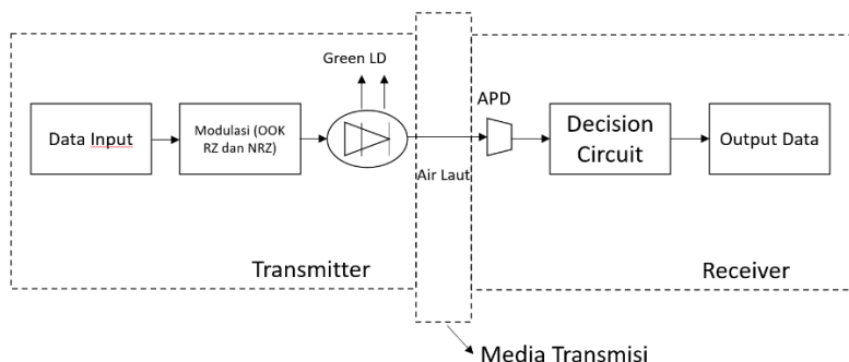
Gambar 3.2 Blok Diagram.
