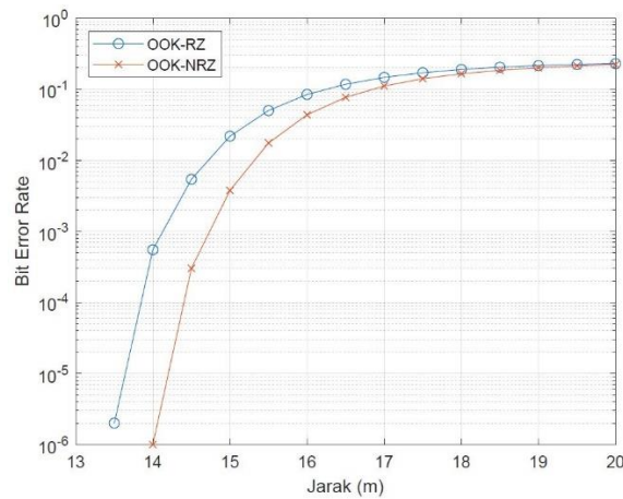
Gambar 4.2 Grafik perbandingan Jarak terhadap BER pada modulasi OOK RZ dan NRZ dengan jenis air Clean Ocean Water .
