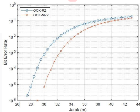
Gambar 4.3 Grafik perbandingan Jarak terhadap BER pada modulasi OOK RZ dan NRZ dengan jenis air Pure Sea Water .
