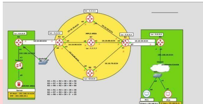
Gambar 4.5 Skenario Spoofing MPLSVpn pada CE-PE
