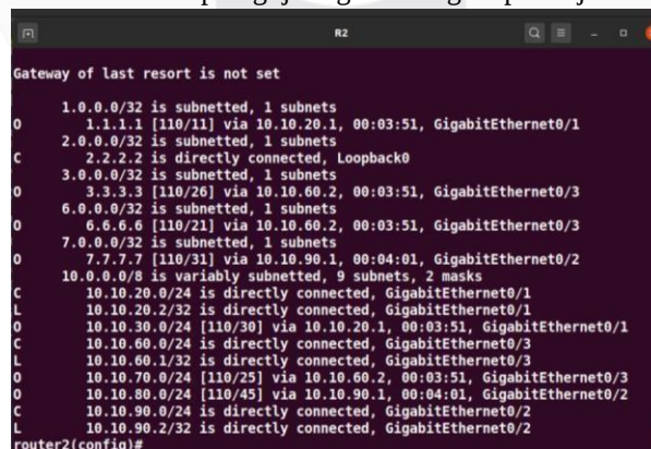
Gambar 4.10 Tabel routing sisi PE sebelum dilakukan ipv4 injection
