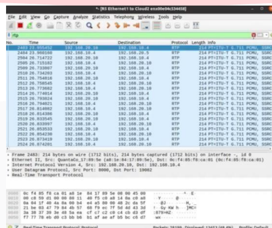
Gambar 4.18 Sniffing Komunikasi Voip
