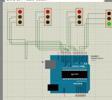
Gambar 4 Rangkaian Lampu Lalu Lintas.
