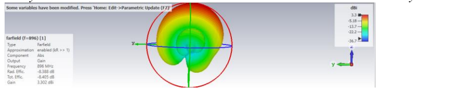
Gambar g. Gain Antena Array 1x4
