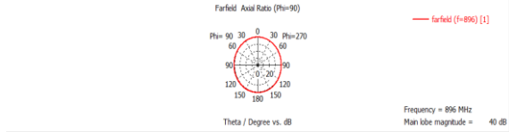
Gambar f. Polarisasi Antena Array 1x4
