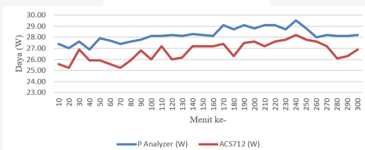
Gambar 9 Grafik perbandingan Daya dengan SMA dan FLC
