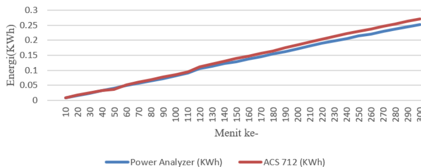
Gambar 7 Grafik Perbandingan kWh dengan SMA
