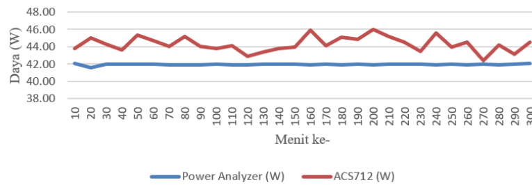
Gambar 6 Grafik perbandingan daya dengan SMA
