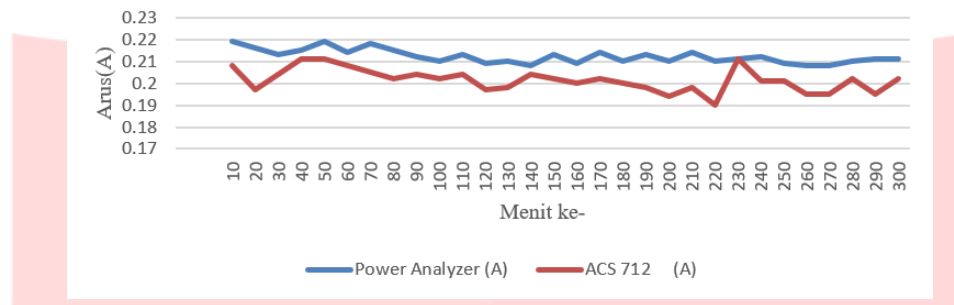
Gambar 8 Grafik perbandingan Arus dengan SMA dan FLC
