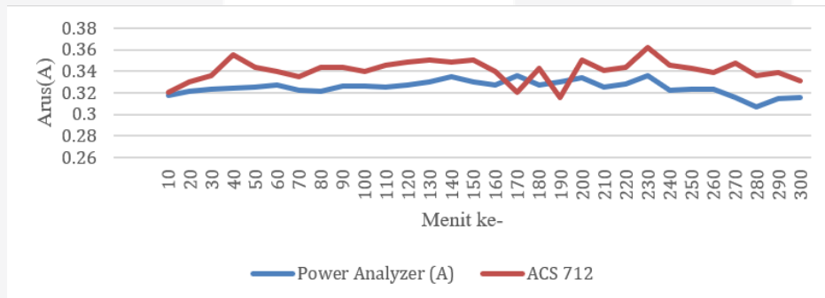
Gambar 5 Grafik Perbandingan Arus dengan SMA
