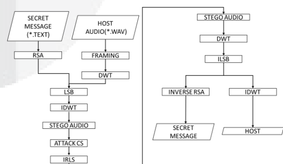
Gambar 2.2 Diagram Blok Sistem
