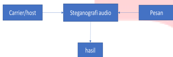
Gambar 2.1 proses steganografi
