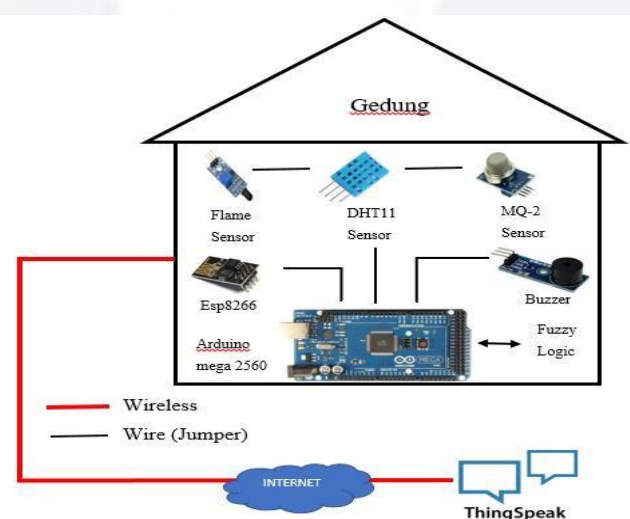
Gambar 3.1 Desain sistem.
